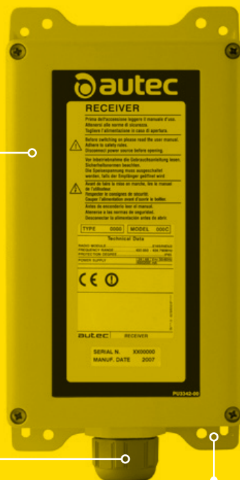
Приемник
